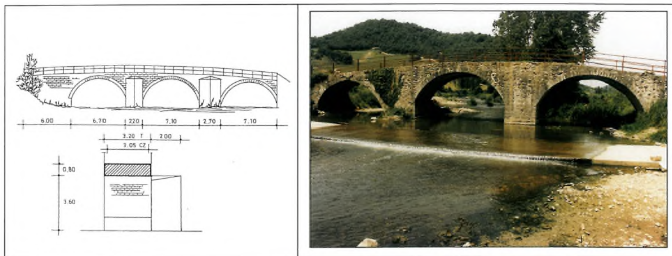
Figura 83.- Croquis y aspecto actual del puente de Ripa, sobre el Ulzama. Archivo Institución Príncipe de Viana. Dirección de Patrimonio Histórico.
