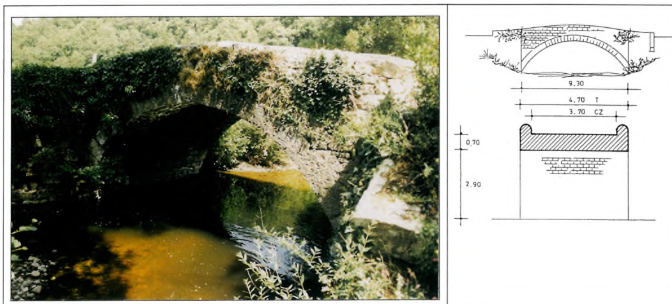
Figura 84.- Puente de Francia sobre el río Mediano, en Etulain. Archivo Institución Príncipe de Viana. Dirección de Patrimonio Histórico.
